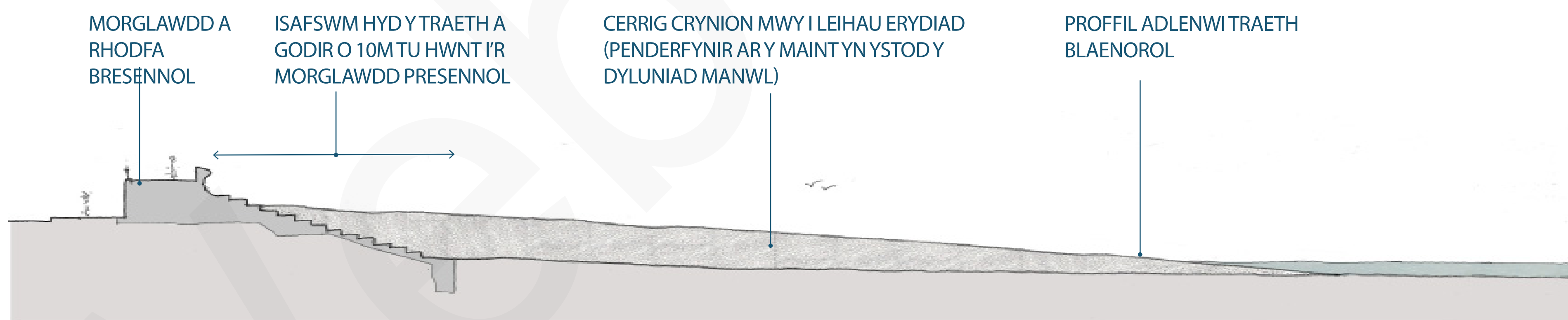
UCHOD: ADRAN AMLINELLLOL YN EDRYCH AM Y DWYRAIN, YN DANGOS Y PROFFIL TRAETH PRESENNOL AC ARFAETHEDIG
