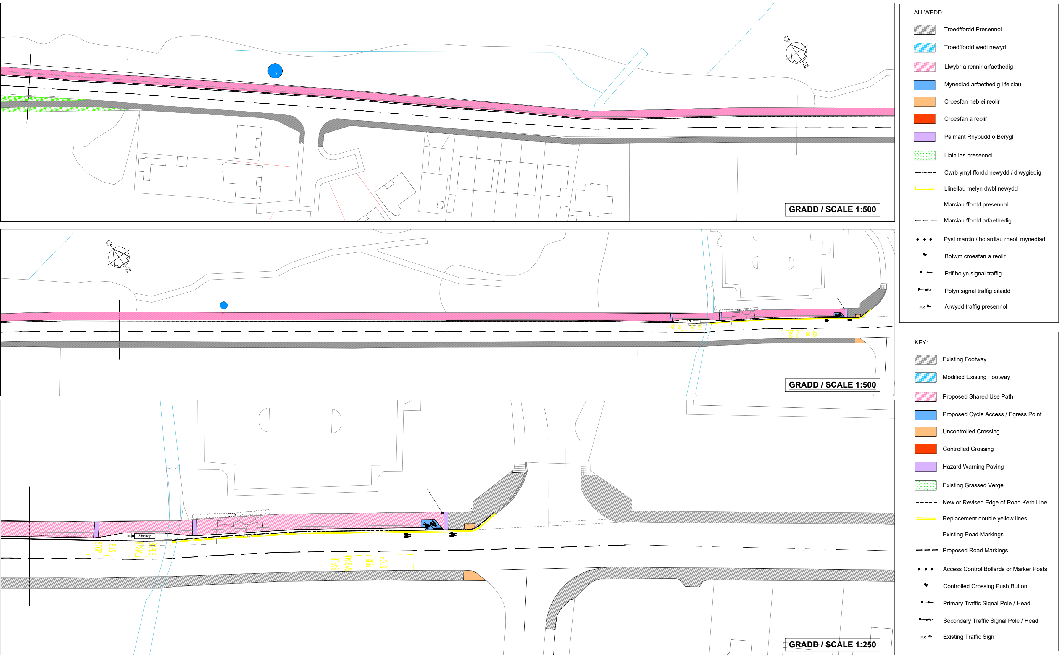
CYNLLUN 2 - Ffordd Llandudno a Coleg Llandrillo DRAWING 2 - LLANDUDNO ROAD AND COLEG LLANDRILLO
